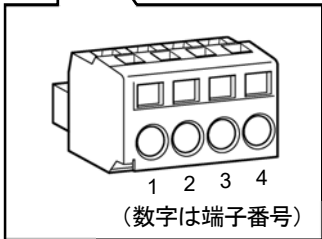
リモート接続用端子台
